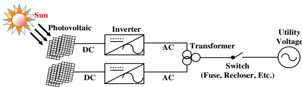
Fig. 7. PV system.
